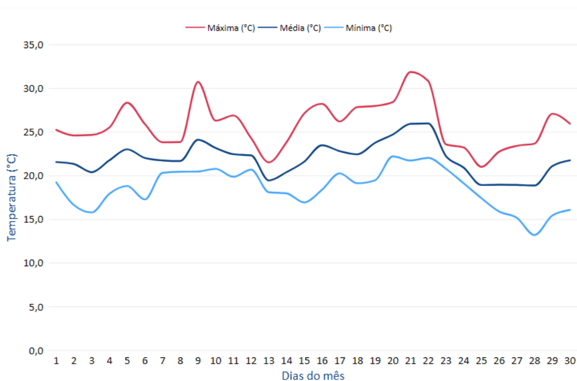
Figura 2. Temperatura máxima, média e mínima diária do mês de setembro de 2025 registradas em Campos dos Goytacazes – RJ.
