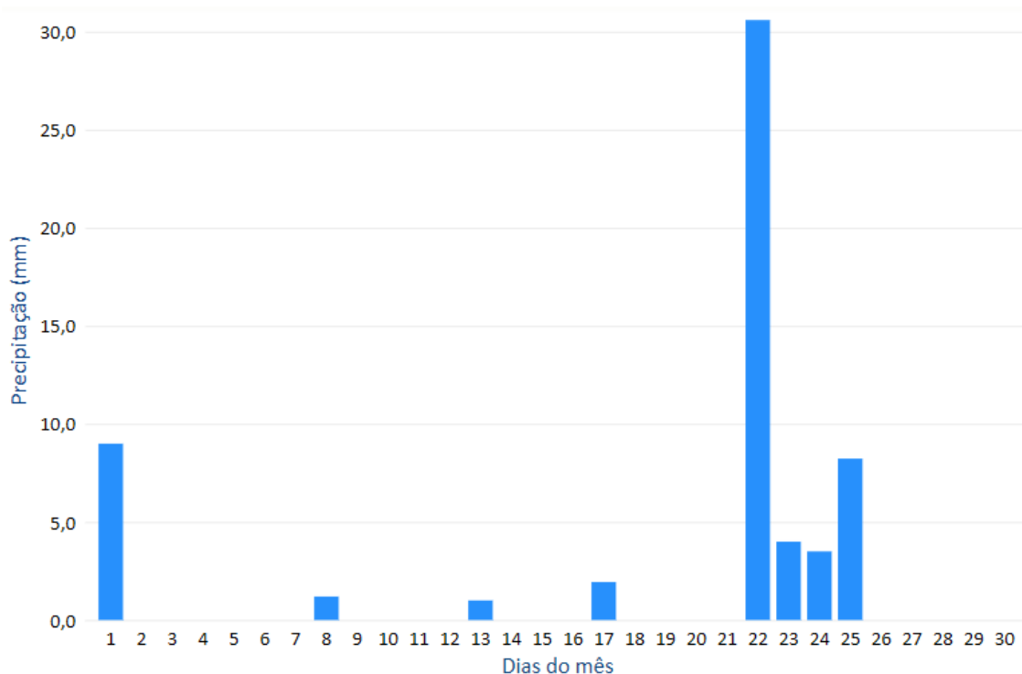
Figura 1. Precipitação diária do mês de setembro de 2025 registrada em Campos dos Goytacazes – RJ.
